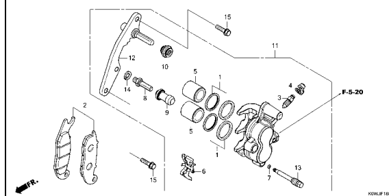
フロントブレーキキャリパー
