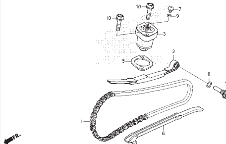
E-5 CAM CHAIN/TENSIONER
