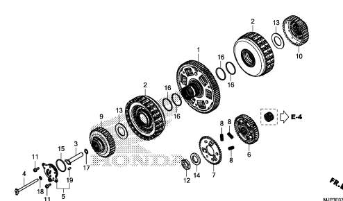
CLUTCH(CRF1000D)
