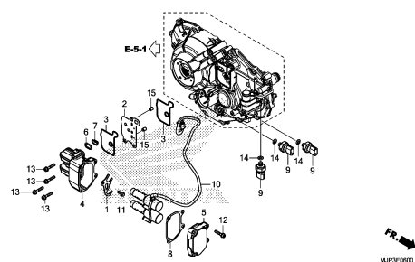
LINEAR SOLENOID
