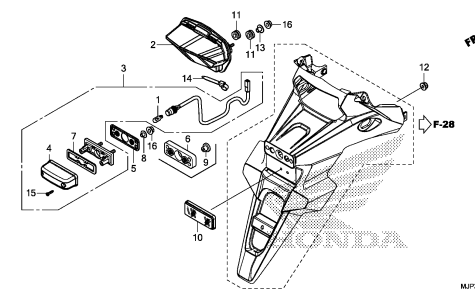
TAILLIGHT/LICENSE LIGHT
