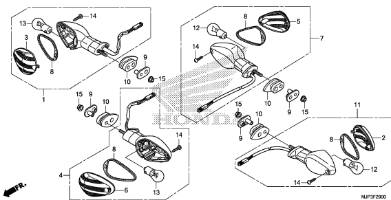
WINKER(CRF1000)
