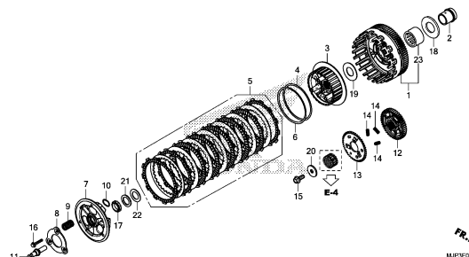
CLUTCH(CRF1000/CRF1000A)
