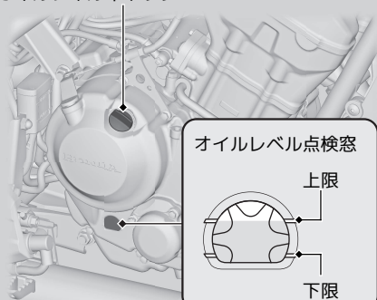
オイルフィルキャップ
