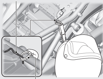
ヘルメットホルダーワイヤー
