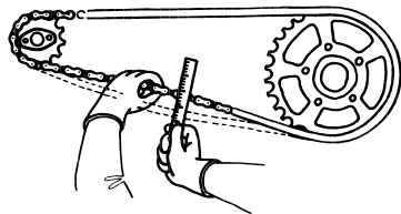
ドライブチェーンの緩み(たるみ)
