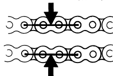
ドライブチェーンの緩み(たるみ)
