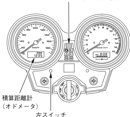
イモビライザーシステム (HISS) 表示灯
