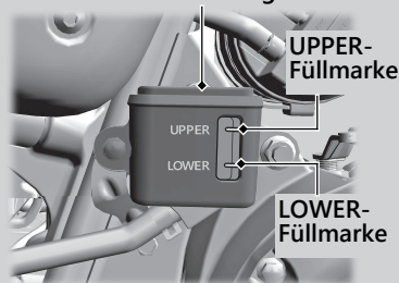
Hinten Hinterradbremssflüssigkeitsbehälter
