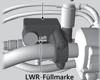
Vorn Vorderradbremssflüssigkeitsbehälter
